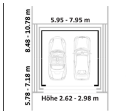
Grundrissvarianten
